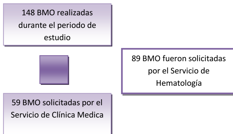
GRAFICO Nº1: ALGORITMO DE FLUJO DE INCORPORACION DE PACIENTES AL ESTUDIO
