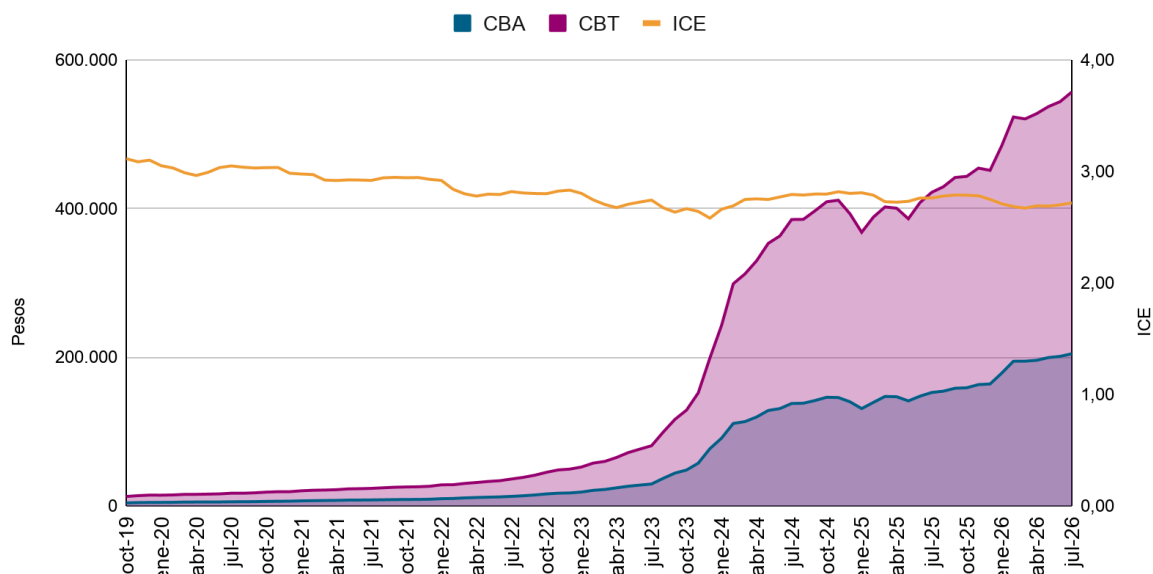
Figura 2. Canasta Básica Alimentaria, Canasta Básica Total (general) por adulto equivalente e Inversa del Coeficiente de Engel. Ciudad de Rosario. Octubre 2019 - julio 2026.
