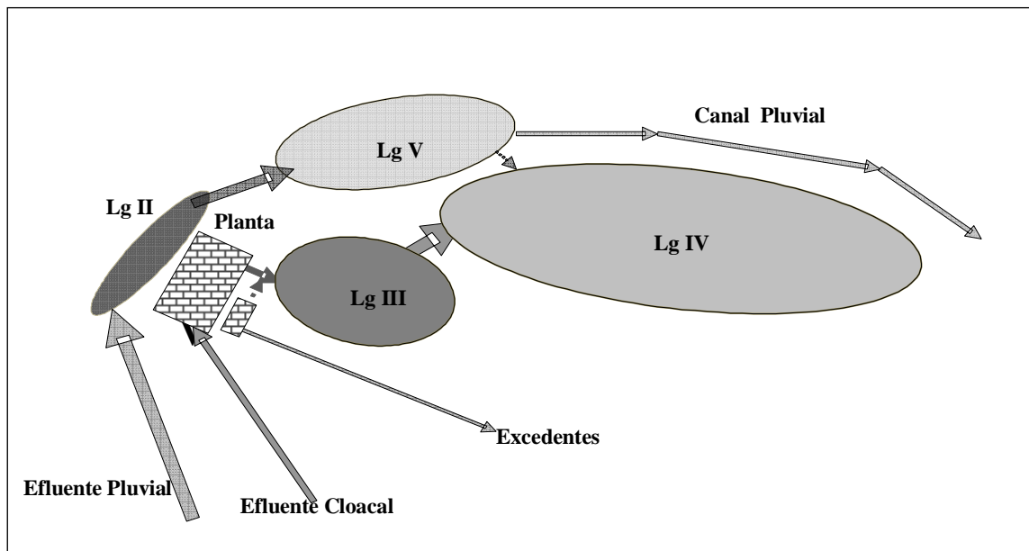
Figura 5. Esquema de componentes e interconexiones superficiales para uno de los escenarios de análisis (Ref. Alternativa 21).
