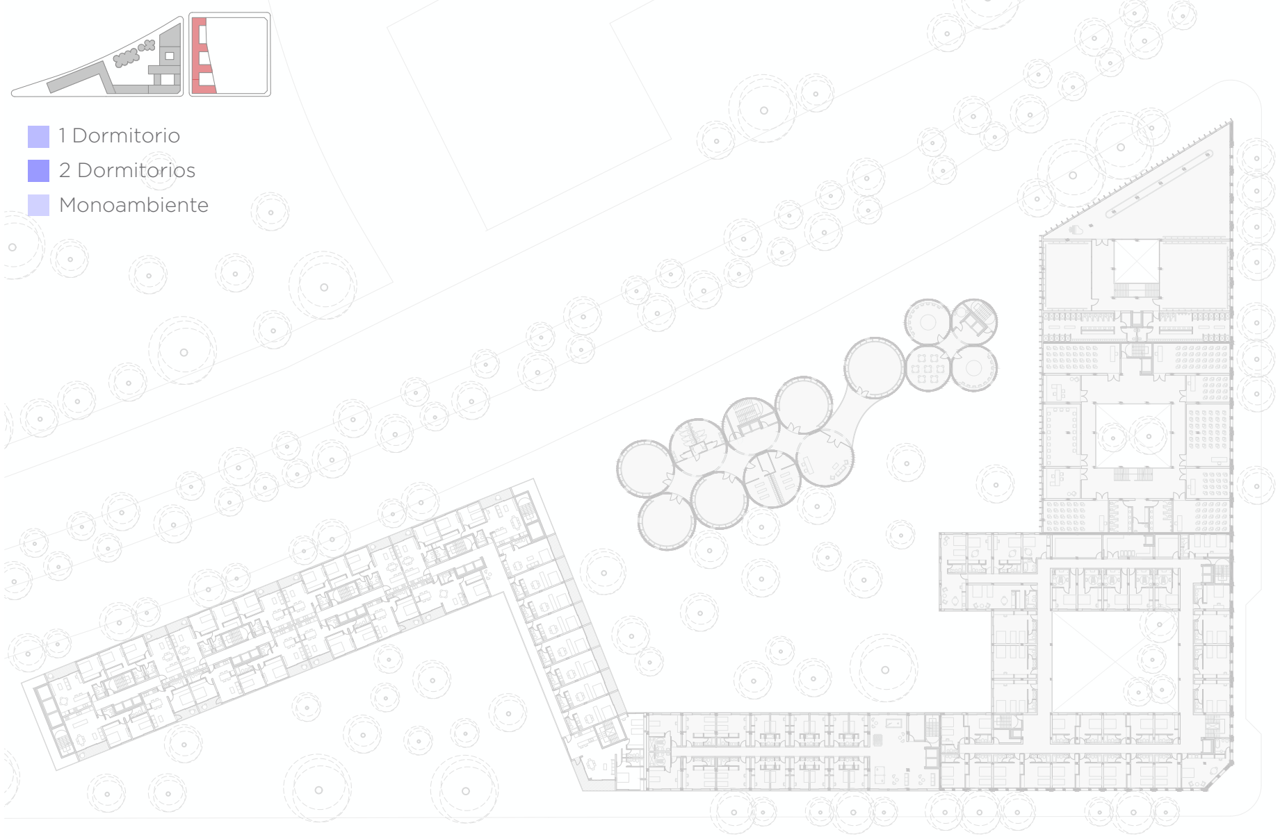
MANZANA 55 - VIVIENDAS - PLANTA TIPO
