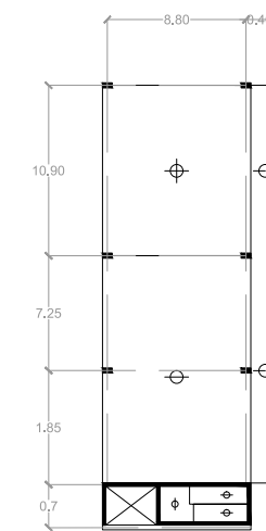
Estructura s/ 2º piso
