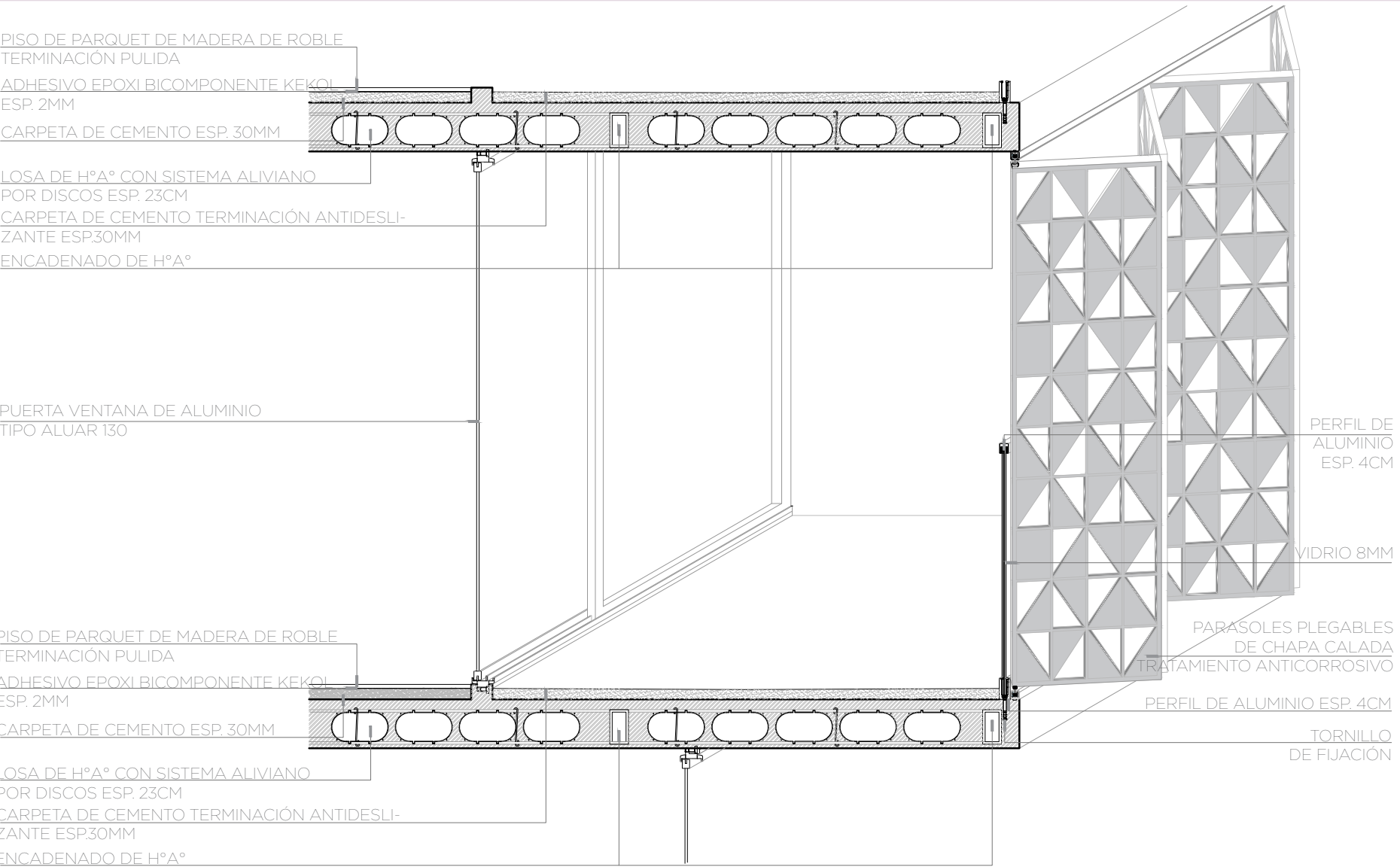
Imagen: Detalle Escala 1:25. Fuente: Autoría propia.
