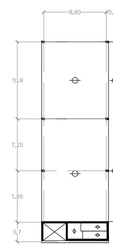
Estructura s/ 3º, 4º, 5º, 6º, 7º Y 8º piso
