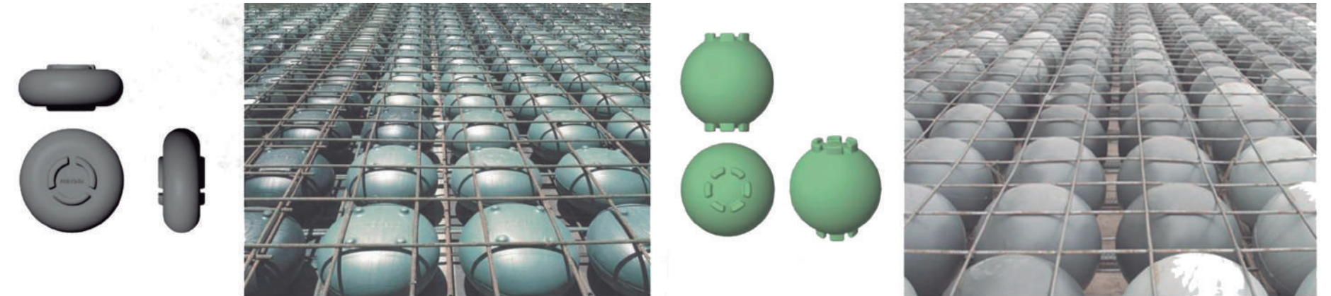
Imagen: Losas Aliviandas con discos (izquierda) y con esferas (derecha) Fuente: Catálogo de losas PreNova.
