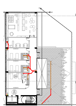
Planta 2° Piso
