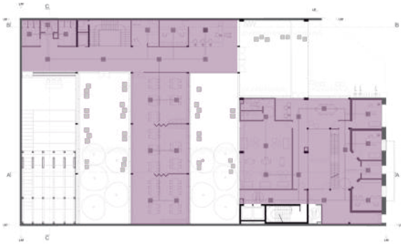
Planta Baja
