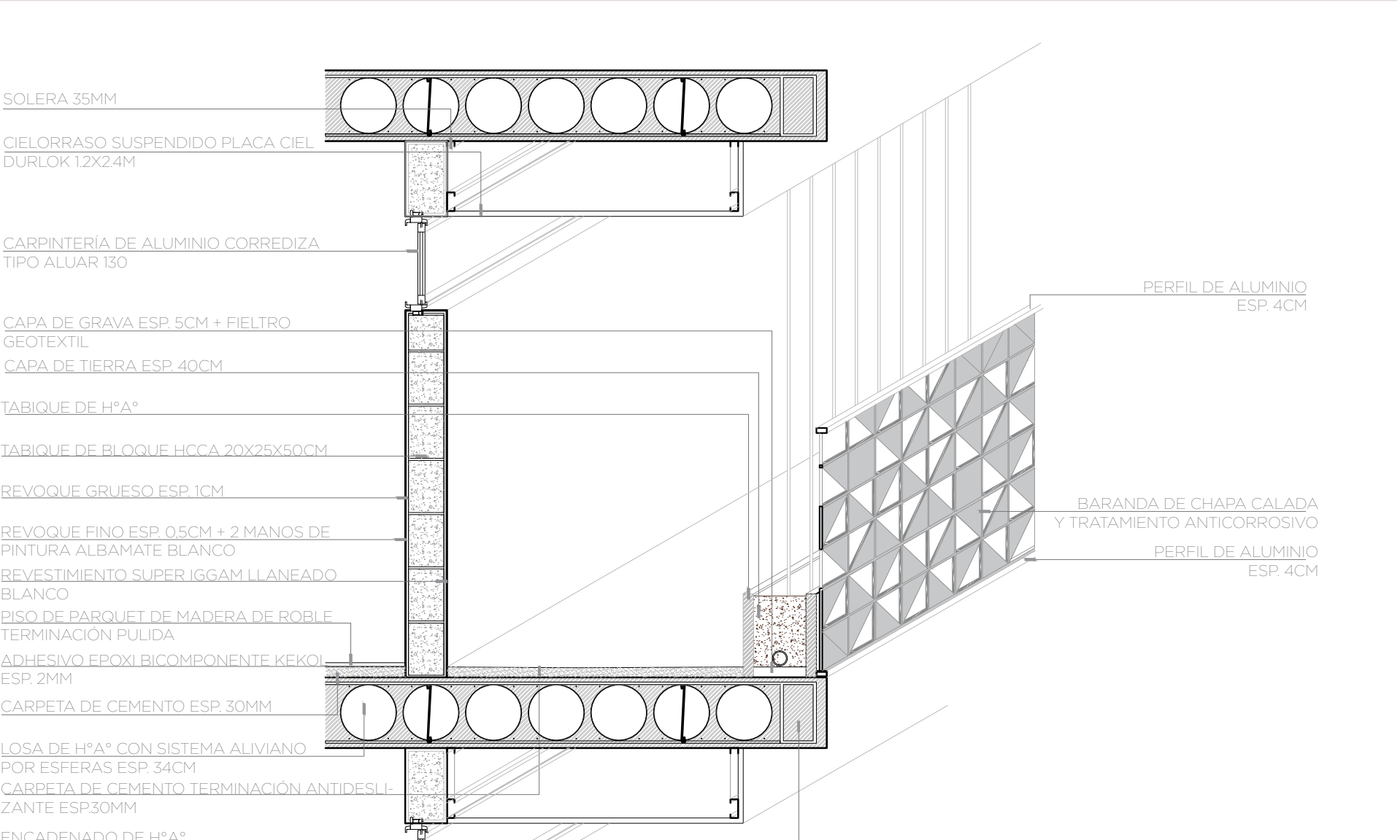
Imagen: Detalle Escala 1:25. Fuente: Autoría propia.
