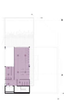
Planta 10° Piso
