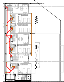
Planta 3° y 4° Piso
