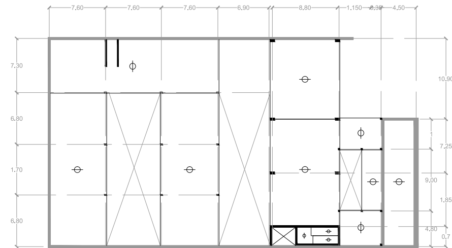
Estructura s/ Planta Baja
