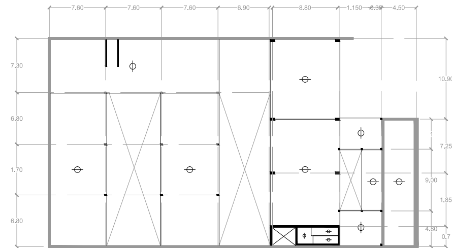
Estructura s/ 1º piso
