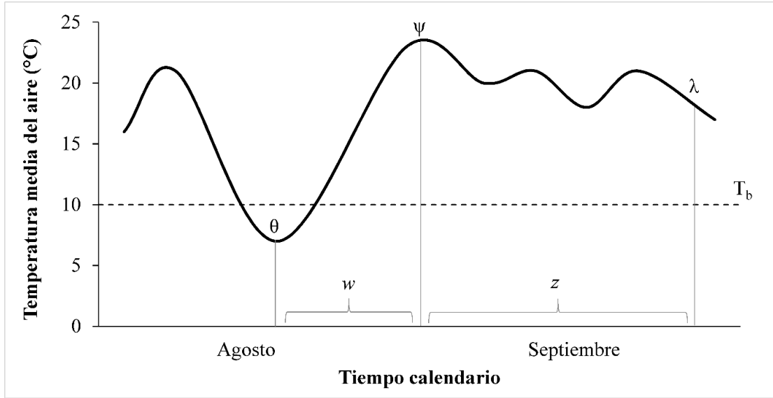
Figura 3.1. Diagrama de la tendencia de la temperatura media diaria en función del tiempo calendario entre fines de agosto y principios de septiembre: \theta es la temperatura mínima del aire por debajo de la T_b (10°C), \psi es la temperatura máxima siguiente, \lambda es la emergencia inicial de las primeras plántulas de E. colona , w es el período de tiempo térmico acumulado entre \theta y \psi , y z es aquel entre \psi y \lambda .
