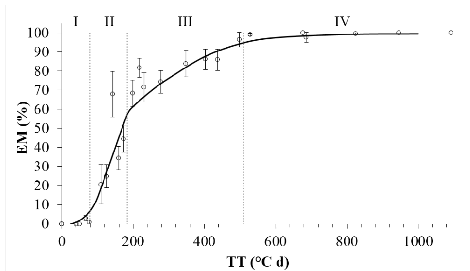
Figura 3.4. Tendencia de emergencia acumulada (EM, %) en función del tiempo térmico expresado en grados día (TT, °C d) en 2014 y 2015. Modelo doble logístico con cuatro etapas: I- fase inicial, II- mayor pendiente, III- pendiente menor y IV- fase final de 'plateau'.
