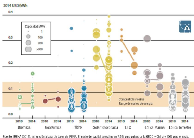
Gráfico 10: Costo de generación total por fuente
