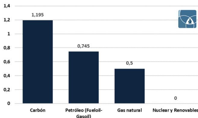
Gráfico 2: Factor de conversión de energía final a emisiones de CO 2 (2014). TC02/Mwh
