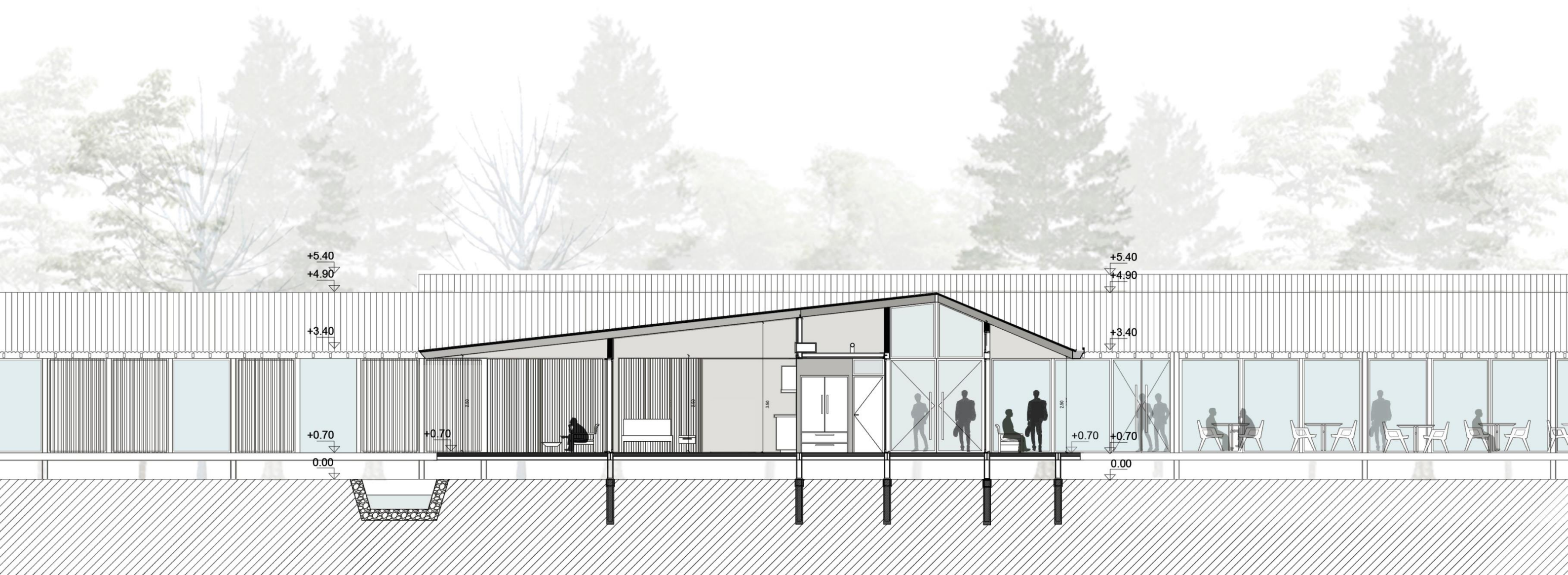
CORTE RESIDENCIAS TEMPORALES
