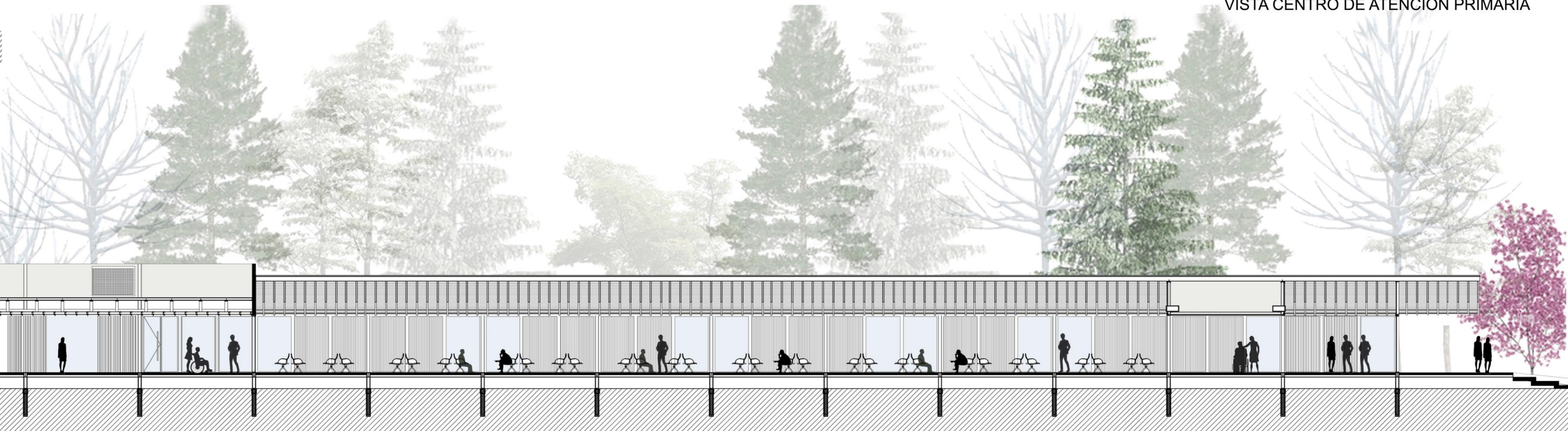
CORTE CENTRO DE ATENCIÓN PRIMARIA
