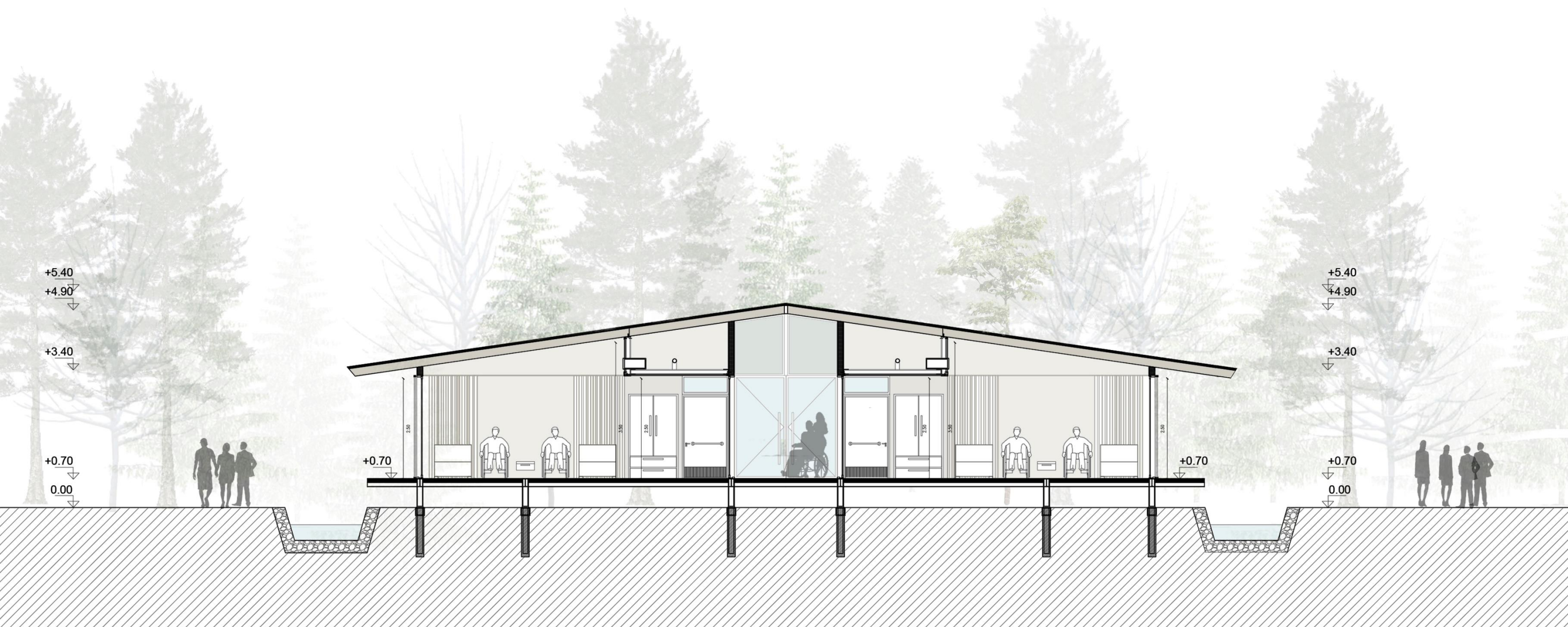
CORTE HABITACIONES INTERNACIÓN
