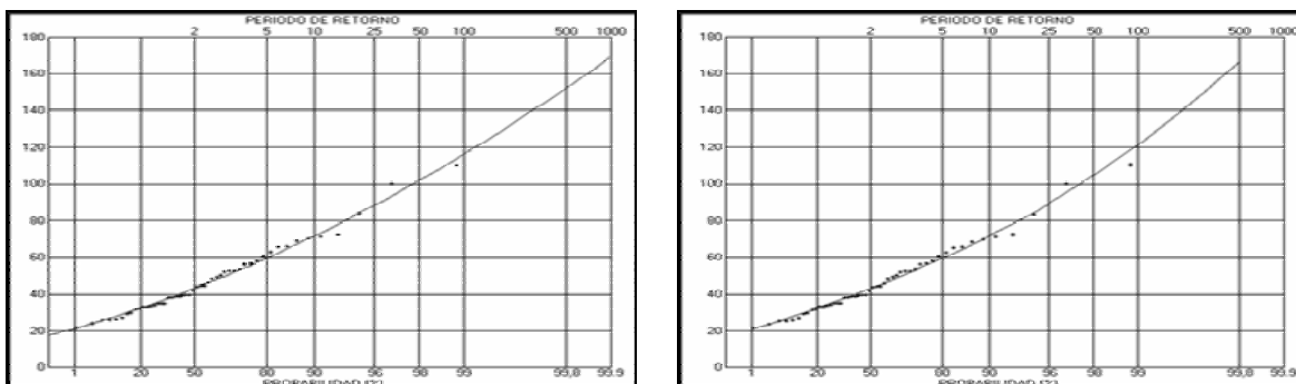
Figura 5. Ajuste de Precipitación Máxima Diaria según SQRT y Valores Extremos Generalizados (GEV).
