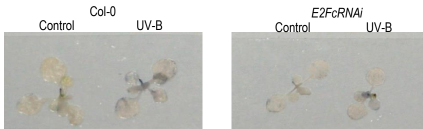
Figura 3.14. Ejemplos representativos de plantas salvajes Col-0 y transgénicas E2FcRNAi de 12 días, teñidas con NBT una vez finalizados los tratamiento con radiación UV-B por 4 horas o en condiciones control. La coloración azul oscuro indica la presencia del anión superóxido. El experimento se realizó por triplicado, obteniéndose resultados similares.
