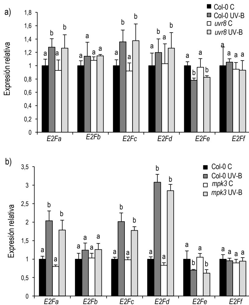
Figura 3.55. Análisis por RT-qPCR de los niveles de los transcritos de cada uno de los E2F , en las hojas #5 de a) las plantas mutantes uvr8 , b) las plantas mutantes mpk3 y las plantas salvajes Col-0 (a y b), sometidas a tratamientos con radiación UV-B o en condiciones control. Las barras representan la expresión promedio relativizada al promedio obtenido para las plantas salvajes en condiciones control. Para la normalización de los datos se utilizó el gen CPK3 . Las barras de error corresponden al error estándar y las distintas letras indican diferencias estadísticamente significativas al aplicar la prueba ANOVA ( p < 0,05 ). Las medidas se realizaron por duplicado, obteniéndose resultados similares.
