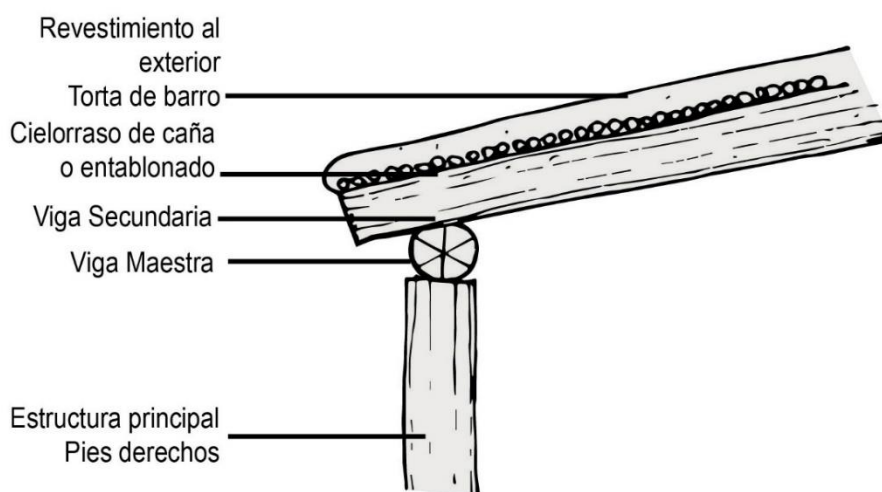
Figura 86. Composición de la Torta de sobre cañas
