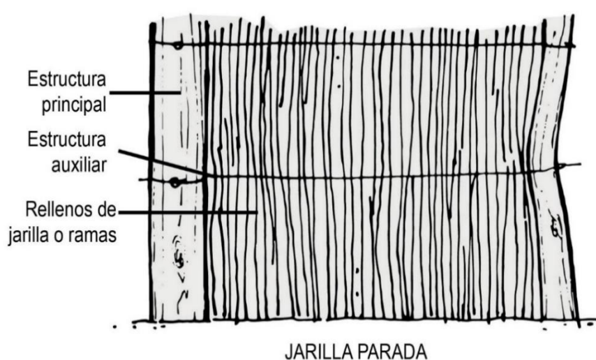
Figura 89. Composición de Jarilla Parada
