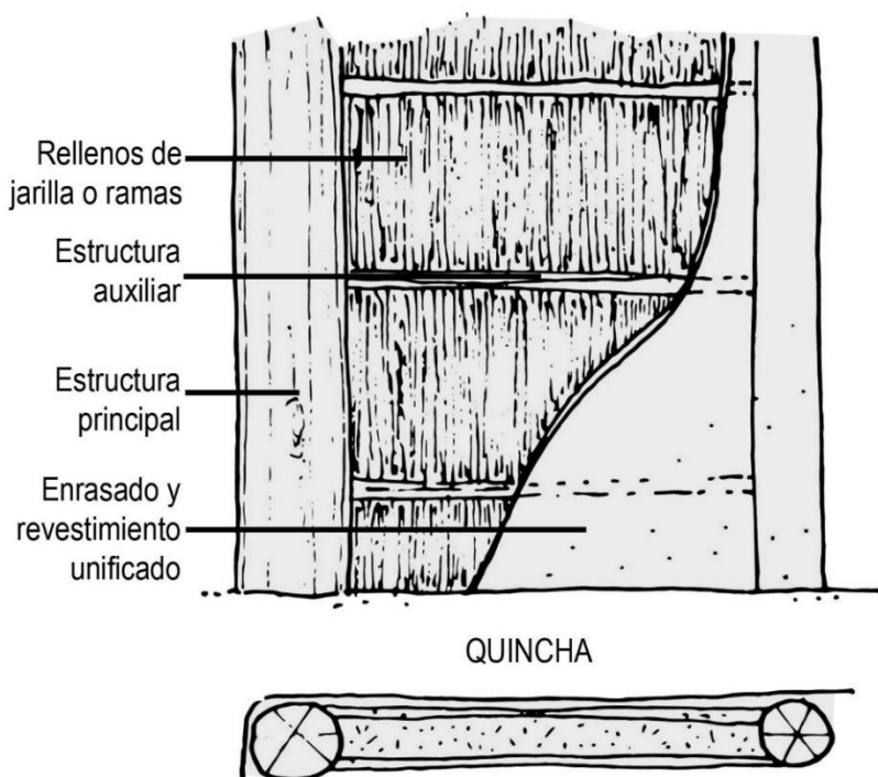
Figura 80. Composición de la quincha en la zona
