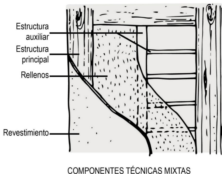
Figura 77. Componentes de las técnicas mixtas
