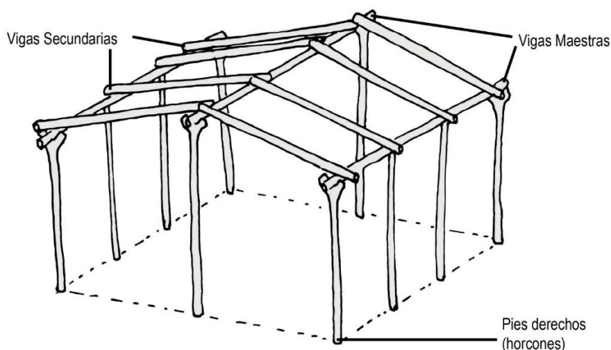
Figura 76. Estructura de madera en sistemas de entramado de la zona
