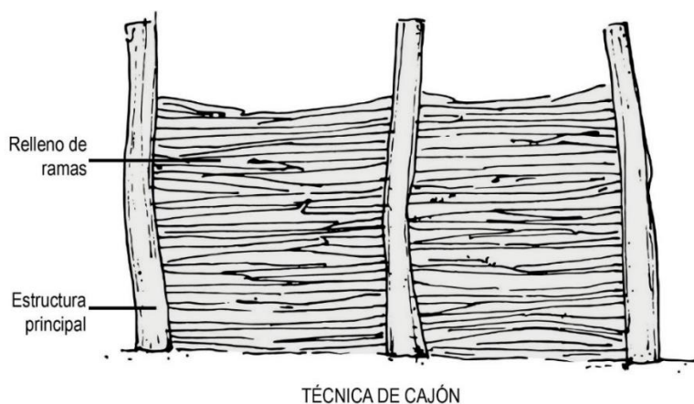
Figura 93. Técnica de cajón
