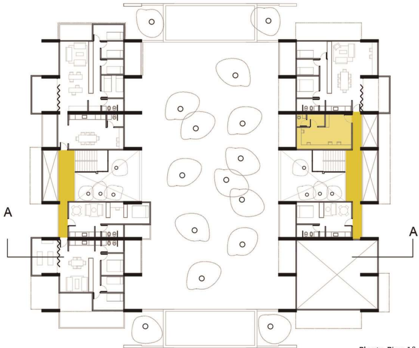
Planta Piso 1º Esc.: 1:250
