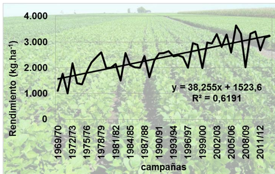
Figura 2: Rendimientos de soja y su tendencia lineal
