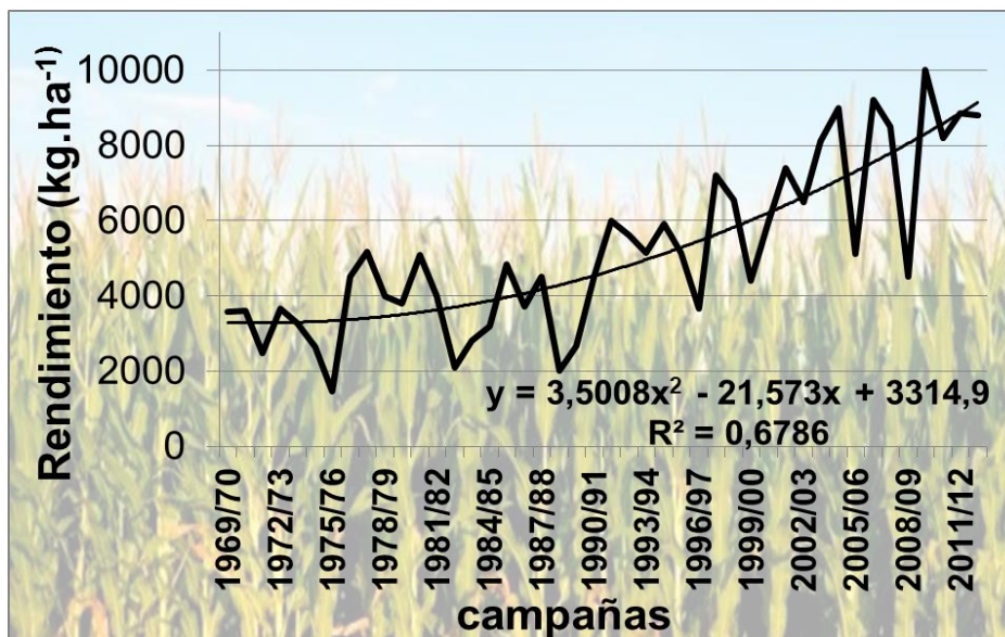
Figura 1: Rendimientos de maíz y su tendencia cuadrática
