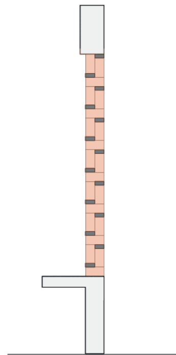
VISTA LATERAL
