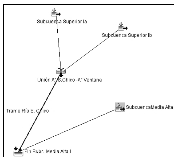
Figura 6. Esquema de control para la simulación - Tormenta del 8 al 10/Nov/2002.
