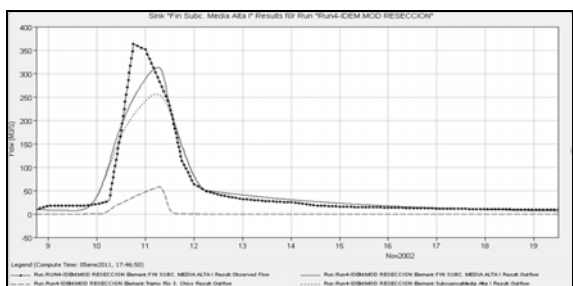
Figura 11. Hidrogramas calculado y observado en RN 35.
