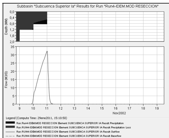
Figura 7. Evento Nov/2002 - Hidrograma en Subcuenca Superior Ia.
