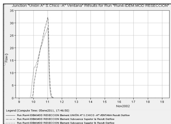
Figura 9. Evento Nov/2002 - Hidrogramas de las Subcuencas Ia y Ib en el punto de unión (Balneario Tornquist).
