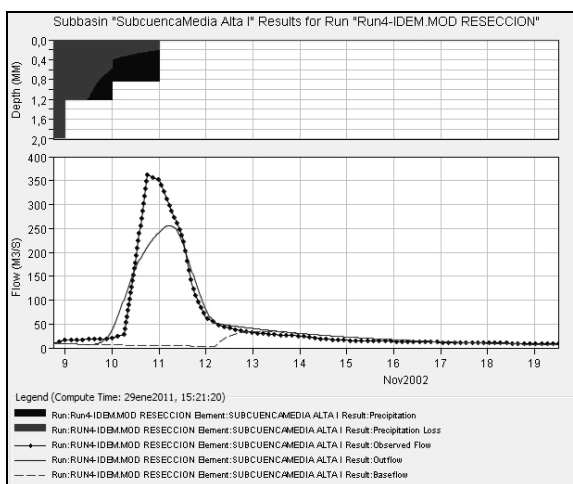
Figura 10. Evento Nov/2002 - Hidrograma de Subcuenca Media Alta I en RN 35.
