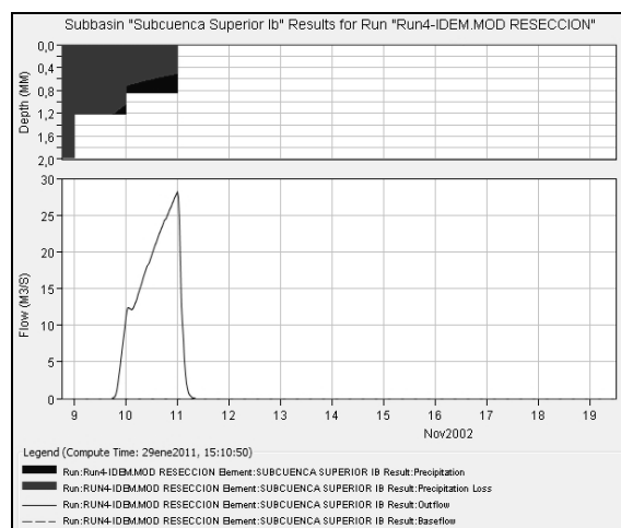
Figura 8. Evento Nov/2002 - Hidrograma en Subcuenca Superior Ib.
