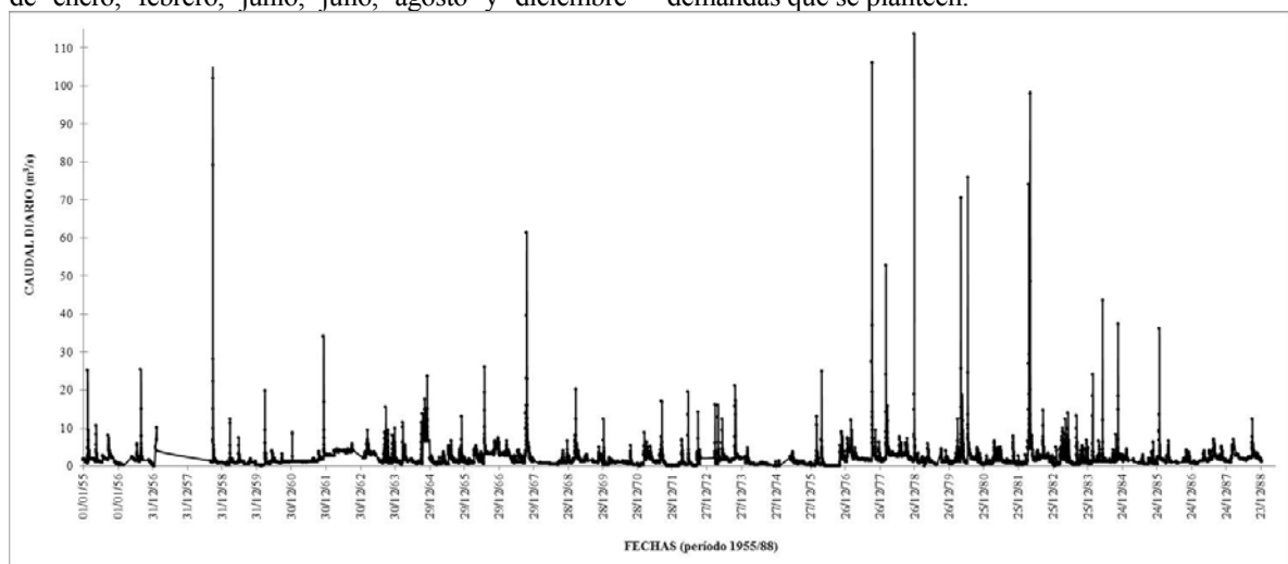
Figura 2. Río Sauce Chico – Estación HL6005-ADA- Serie histórica de caudales diarios – Período 1955/88: 10587 datos.
