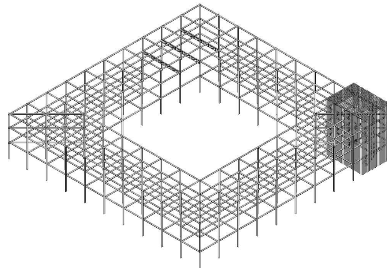
ESQUEMA ESTRUCTURAL PRIMARIO
