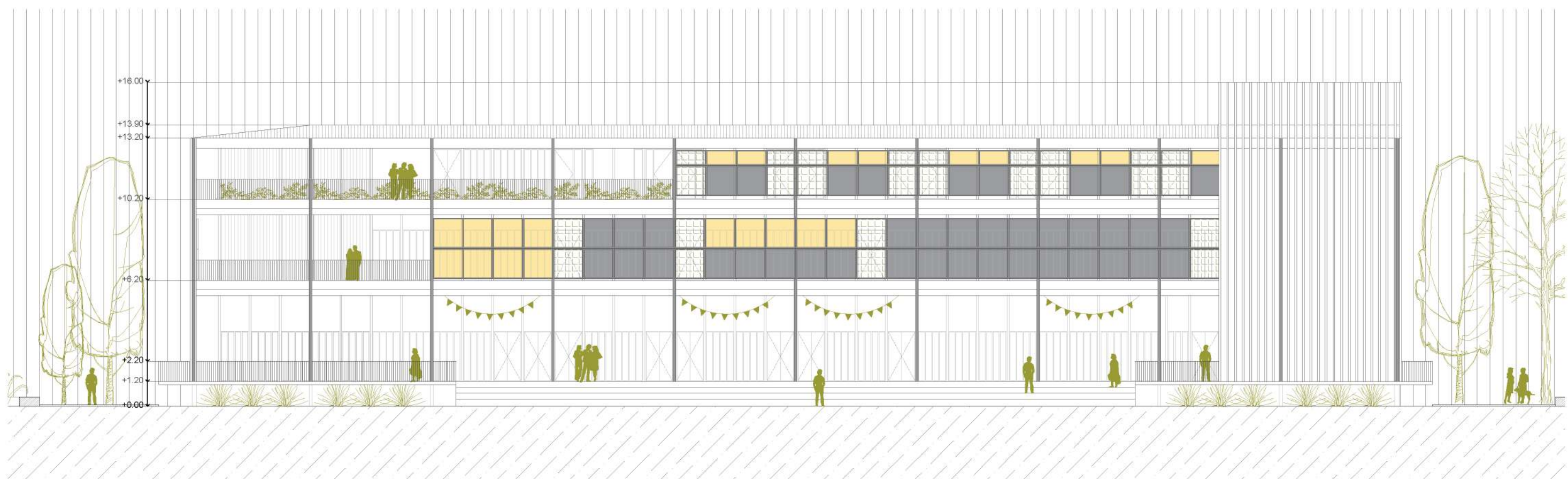
Vista este | ESC 1.200
