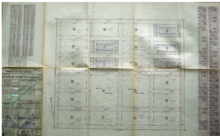
4. Plano de proyecto de loteo para el pueblo de Soldado Maldonado. Departamento de Geodesia y Topografía, 1977. Fuente: Archivos de Catastro de la Provincia de Tucumán. Investigador: Pamela Colombo
