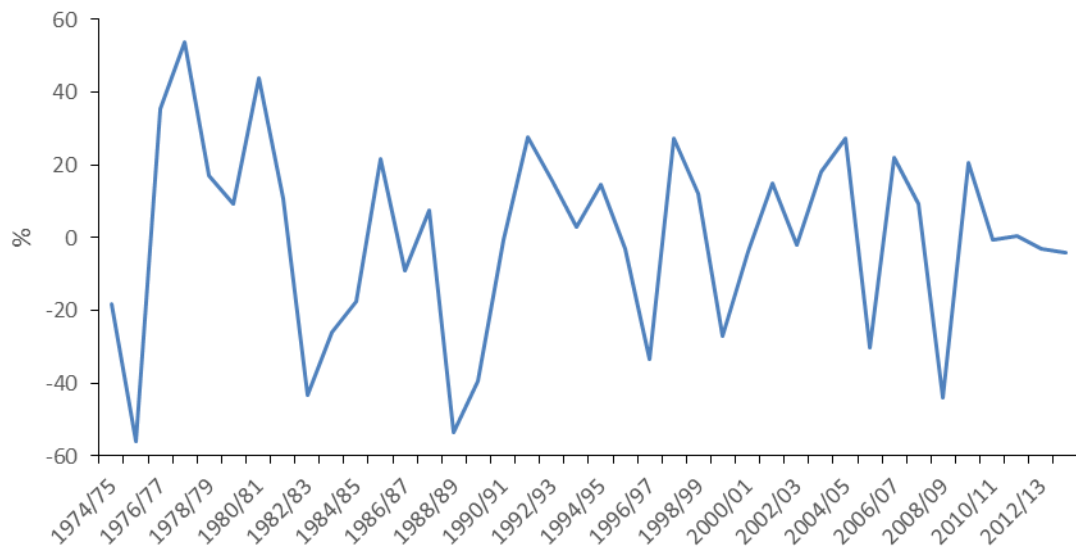
Figura 6: Evolución de la variación porcentual de los rendimientos observados (R) respecto a los rendimientos ajustados (Raj) por un polinomio de segundo grado. Período 1974-2014.
