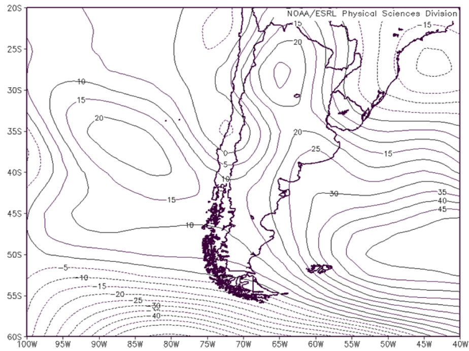
Figura 20: Campo medio de anomalías de altura geopotencial de 1000 hPa. para las mTS del PC2. Campañas: 1996/97; 1999/00; 2005/06 y 2008/09
