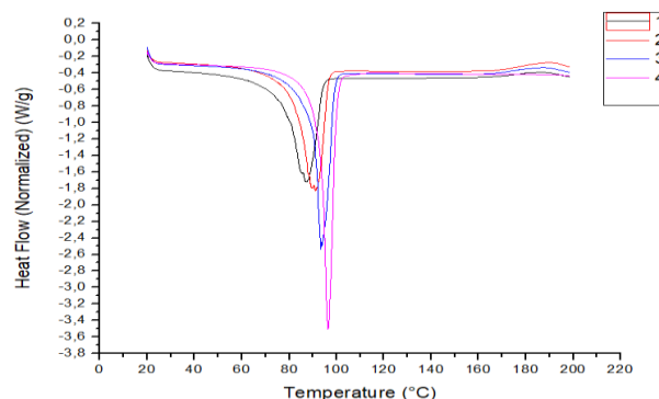
Figura 1. Purificación de lactida con acetato de butilo en DSC El producto de reacción se caracterizó mediante FTIR para corroborar la estructura química del producto obtenido. En la Figura 2 a) se puede observar la presencia del pico en 3000 cm -1 C-H, 1750 cm -1 C=O, 1150 cm -1 C-O, característicos del PLA. Por otra parte, en la Fig. 2 b) se observan las transiciones de fase típicas del PLA 1 , observándose una Tg a 45°C, un pico exotérmico de cristalización en frío a 100°C y la fusión del polímero con picos endotérmicos a 135 y 155°C
