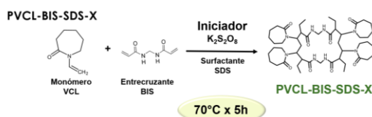
Figura 1. Síntesis de los Ngs de PVCL-BIS.
