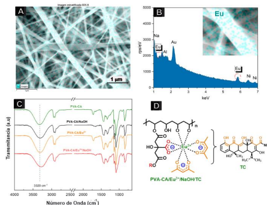
Figura 1. A: SEM, B: Espectro EDS, C: FTIR de las mallas de PVA-CA/ \text{Eu}^{3+} /NaOH y D: Complejo PVA-CA/ \text{Eu}^{3+} /NaOH-TC.
