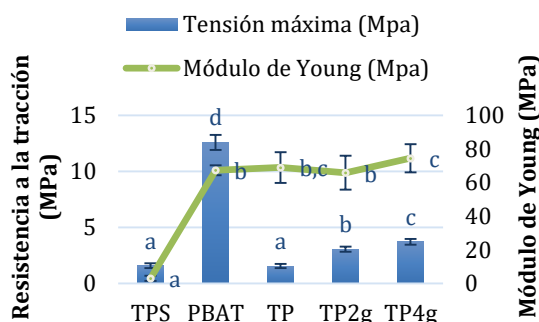
Figura 1. Resistencia a la tracción y Módulo de Young de los films de TPS, PBAT y los sistemas compuestos.
