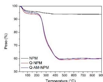
Figura 1. Curvas de TGA de las partículas sintetizadas.
