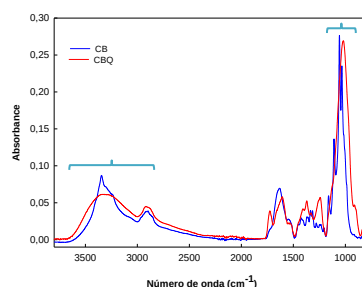
Figura 1. Espectros ATR-FTIR de biofilm de celulosa producido por K. europaeus CIDCA 1143 en presencia (CBQ) o ausencia de quitosano (CB)
