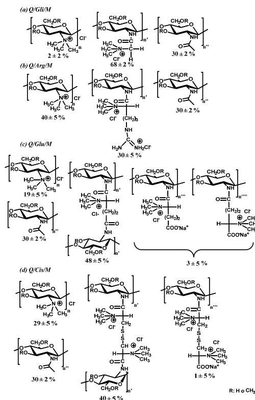
Figura 1. Unidades estructurales presentes en los materiales permitilados.
