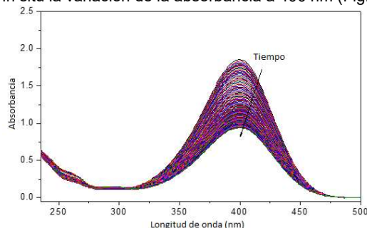
Figura 1. Espectros UV-visible dependientes del tiempo de un experimento representativo utilizando una AuNWs/PF. [\text{NaBH}_4] = 5 \text{ mM} , [\text{PNP}] = 0,1 \text{ mM} .
