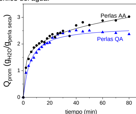
Figura 1. Q(t) para las perlas AA y QA.
