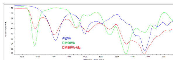
Figura 1. FTIR para DM90VA-Alg, DM90VA, AlgNa.
