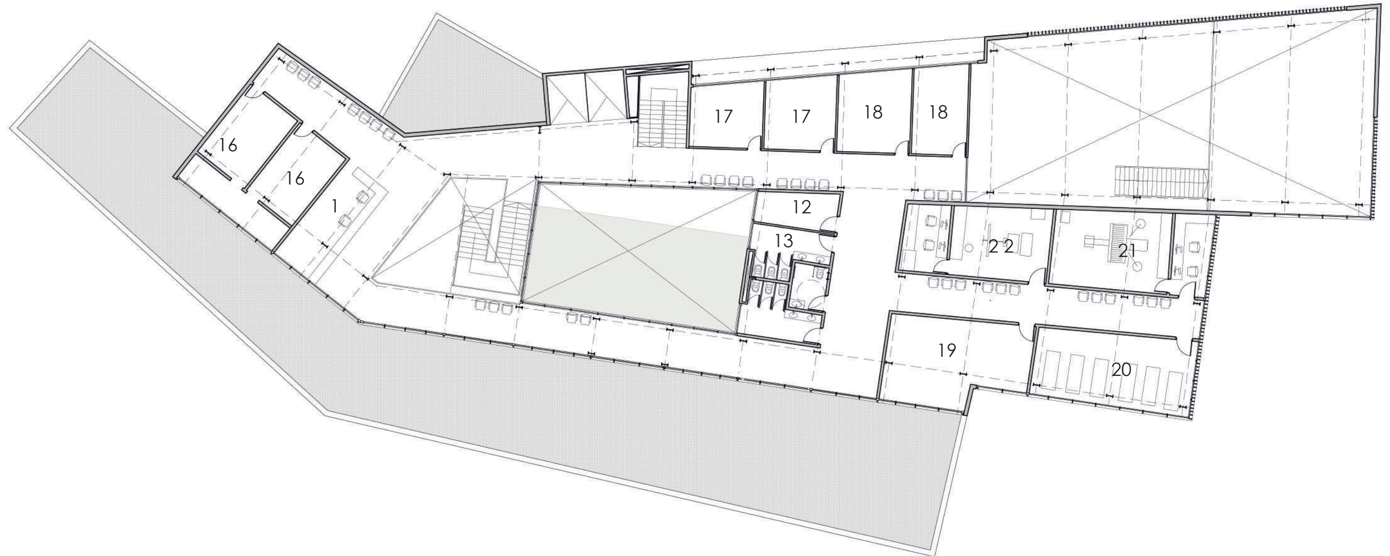
PLANTA 1º PISO
