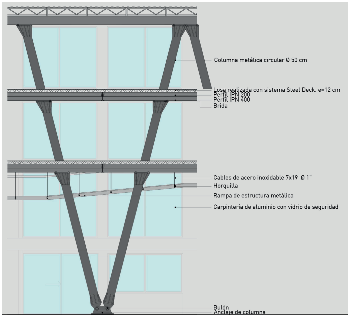
Detalle estructural columna.
