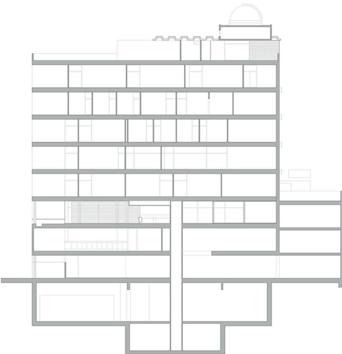
SECCION BIBLIOTECA B-B ESCALA 1: 100
