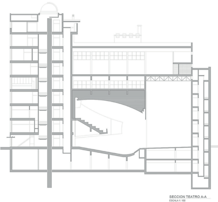
SECCION TEATRO A-A ESCALA 1: 100
