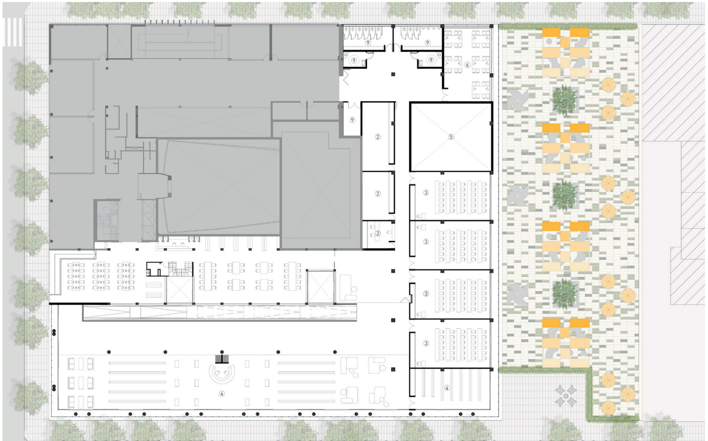
Planta Tercer Piso.
