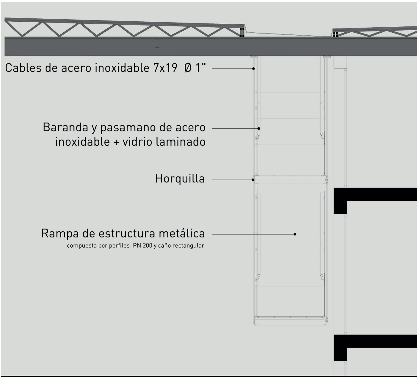
Detalle estructural rampa.
