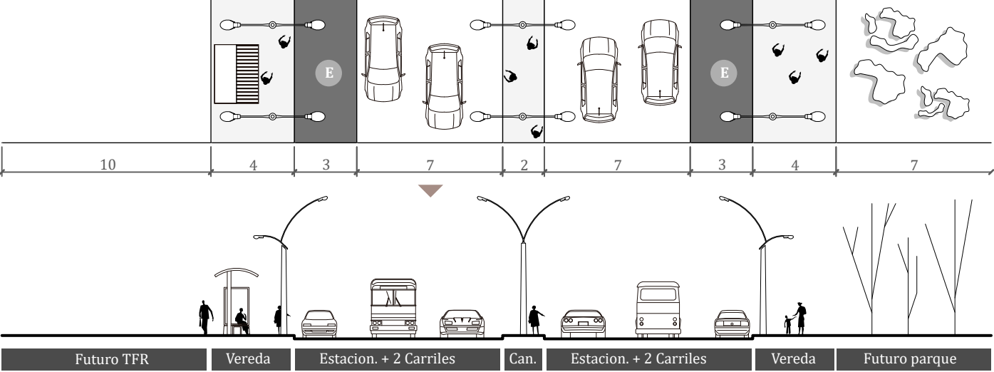
Perfil Nueva Avenida del Eje Metropolitano
