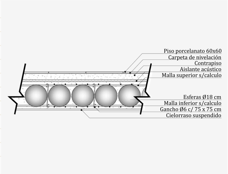
Detalle losa prenova
