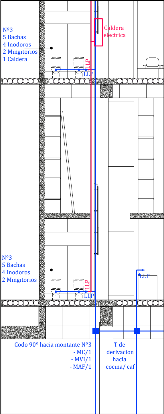
Corte nucleo baños
