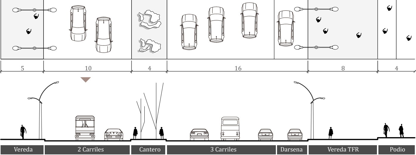
Perfil Avenida Francia
