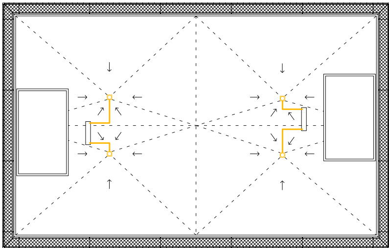
Planta de techo - Desague
