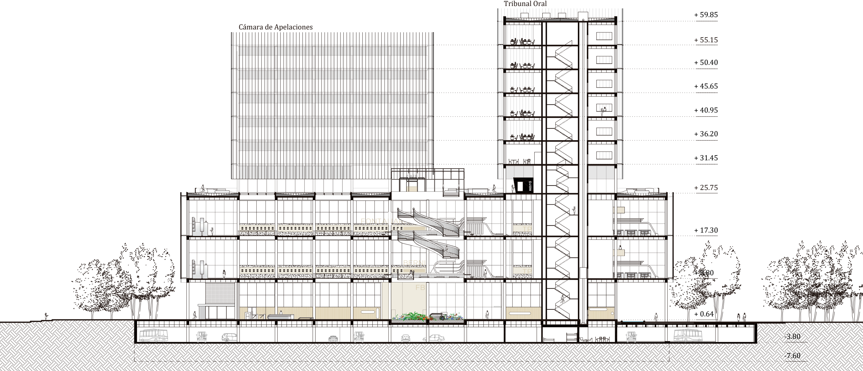
Corte A.A
