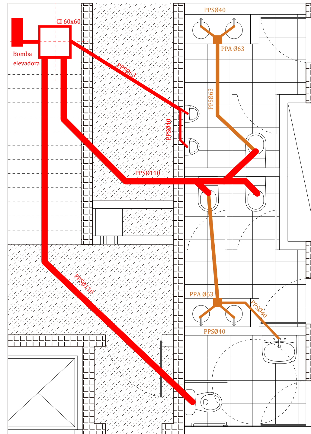
Planta subsuelo núcleo sanitario
