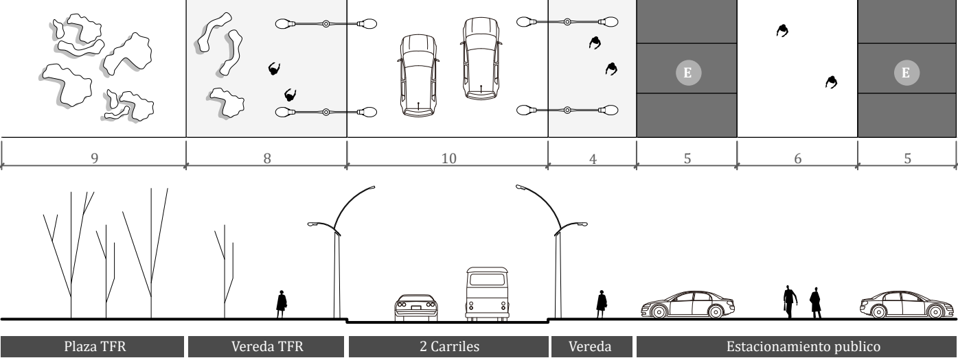
Perfil Nueva calle secundaria
