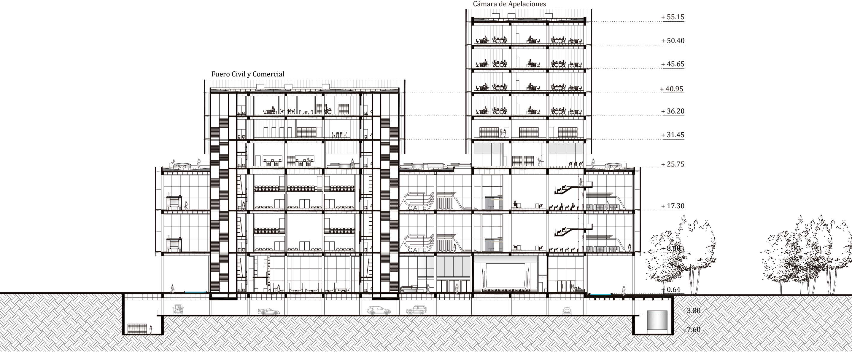
Corte B.B 0 5 10m
