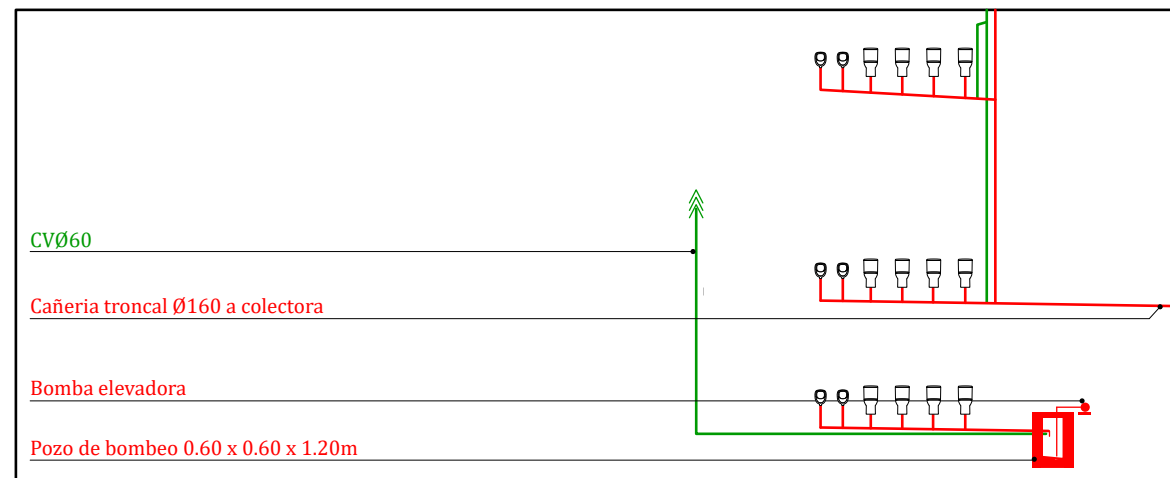
Corte esquema
