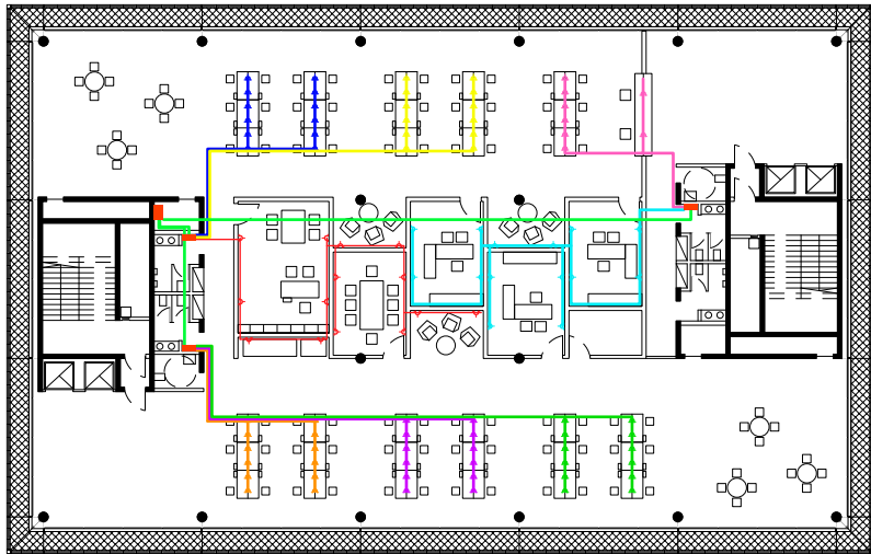
Planta tipo oficinas - Distribución tomacorrientes
