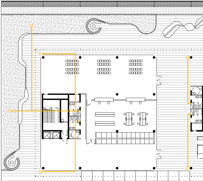
Planta terraza - Distribución de embudos
