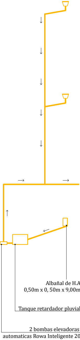
Planta de techo - Desague
