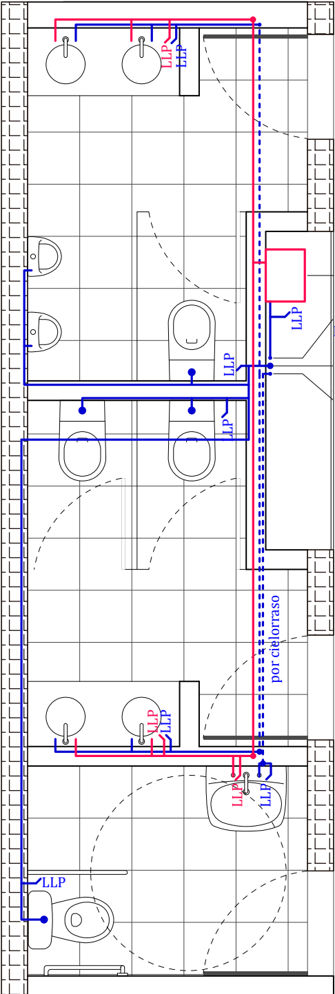
Planta tipo nucleo baños
