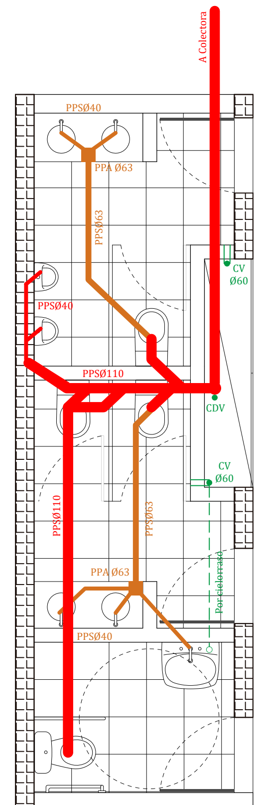
Planta tipo núcleo sanitario
