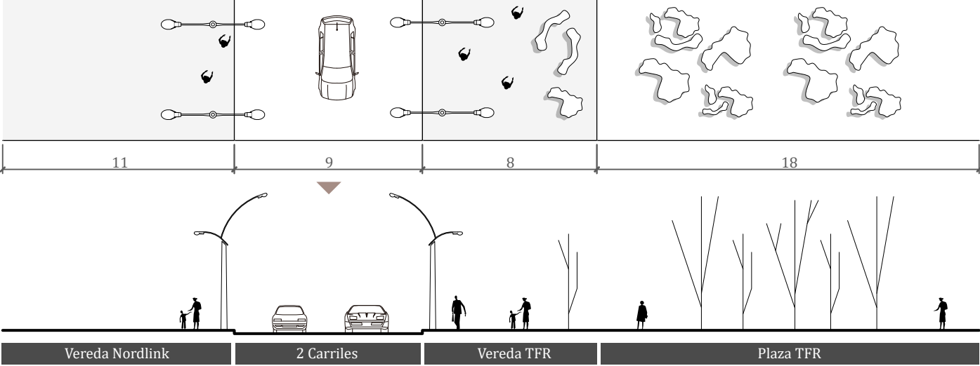
Perfil calle Madres Plaza 25 de Mayo
