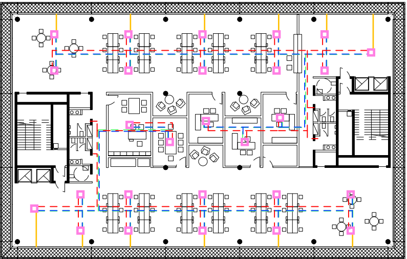
Planta tipo oficinas - Distribución cassette
