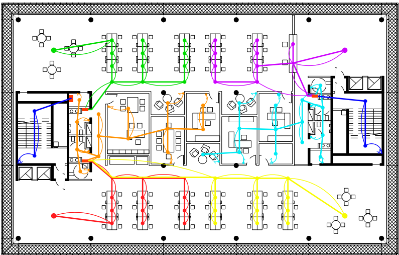
Planta tipo oficinas - Distribución bocas
