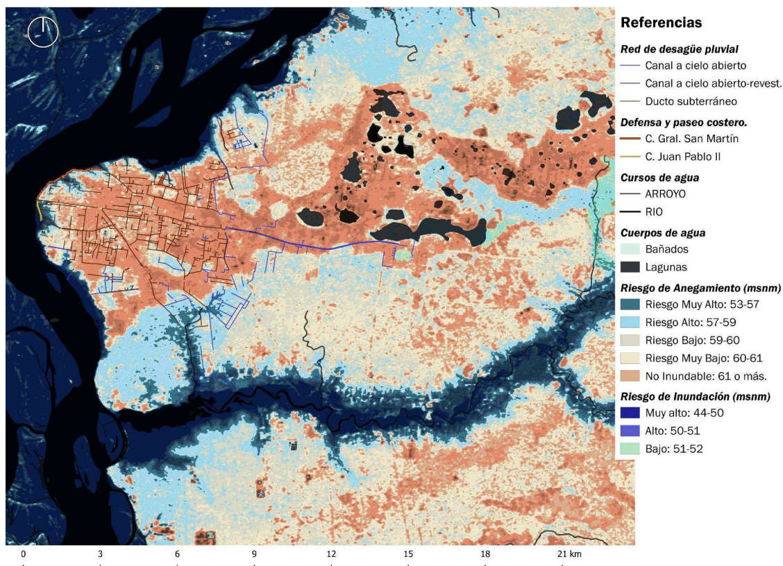
Fig. 3.15: Mapa hipsométrico. Fuente: Rus, 2021.
