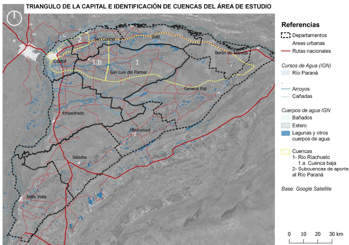
Fig. 3.12: Triángulo de la Capital y cuencas que comprenden el área de estudio. Fuentes: Mapa de recursos hídricos superficiales de la Provincia de Corrientes, ICAA. Giraut et al. (2010), Serra, 2007, MOSP, 1973.
