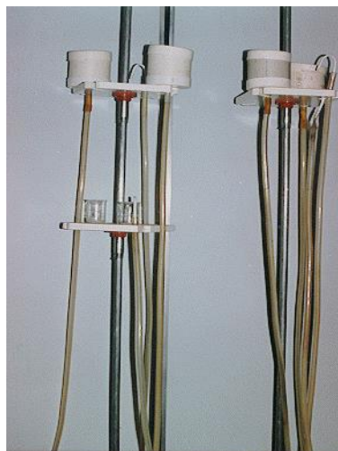
Figura 6. Mesa de tensión para la determinación Capacidad de Campo (CC).
