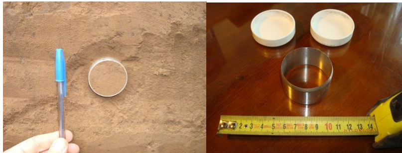
Figura 5. Cilindros de muestreo para la determinación de Capacidad de Campo (CC).
