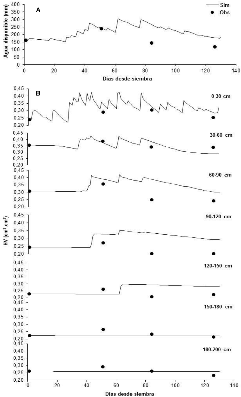
Figura 24. PERGAMINO, campaña 2010-2011. Comparación entre valores observados (puntos) y simulados (líneas continuas). SRGF 1.5, SLRO 91 y SLDR 0.6. A) Agua disponible en mm. B) Humedad volumétrica (HV) en cm 3 .cm -3 por estratos de suelo.
