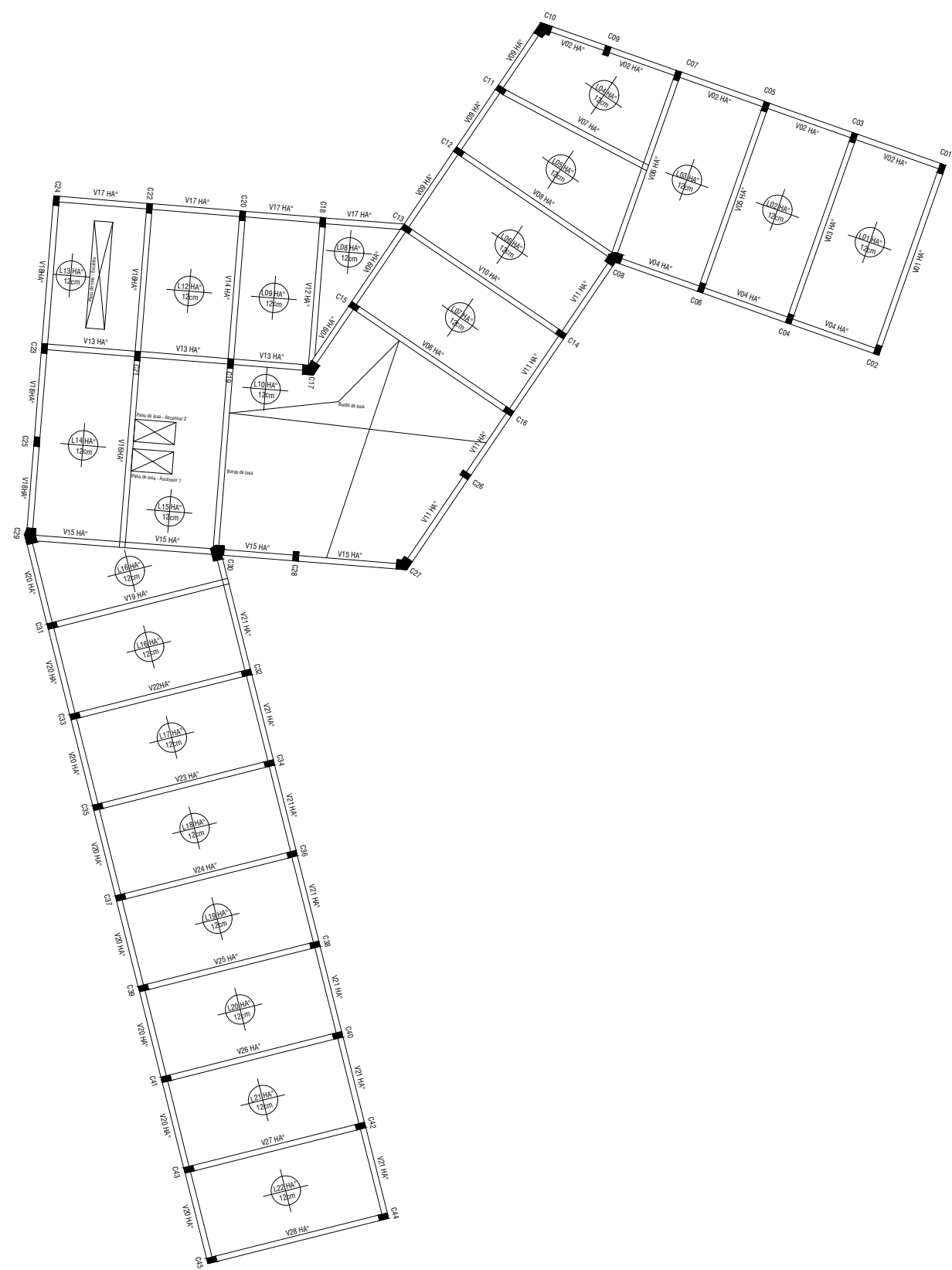
PLANTA DE ESTRUCTURA SOBRE P.B. - Esc. 1.500
