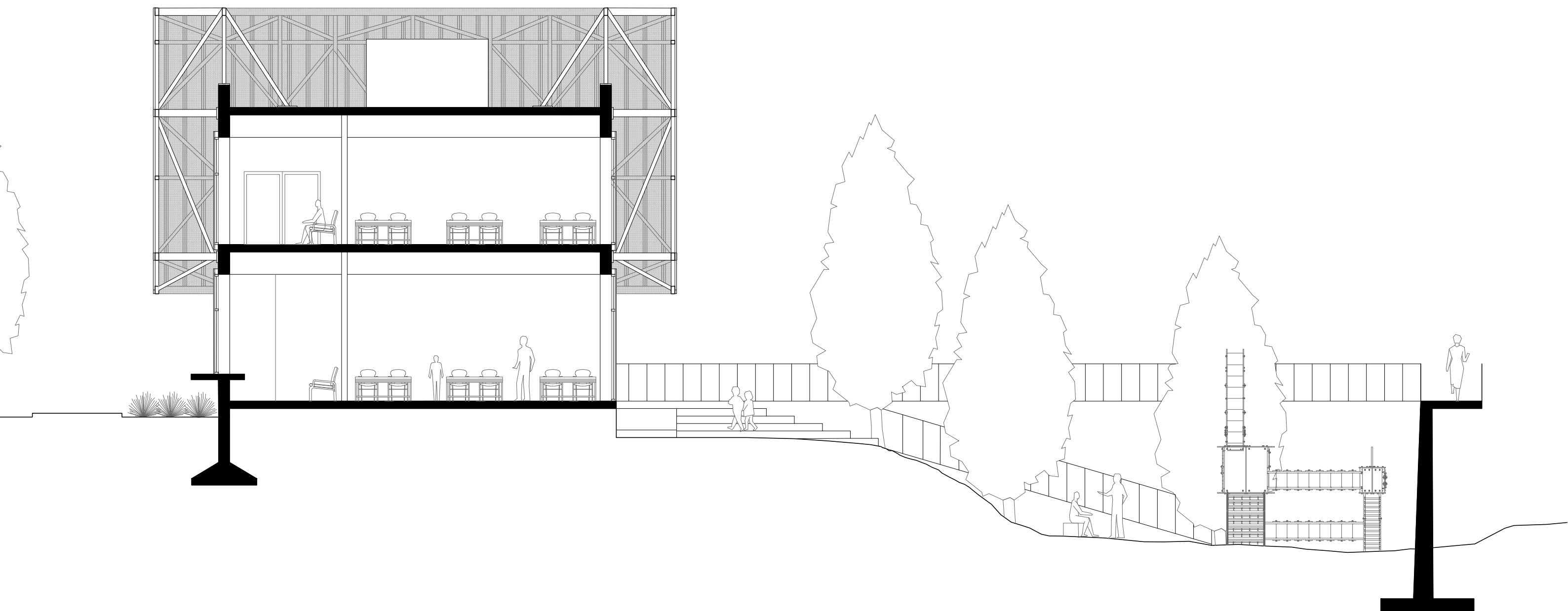
CORTE - CENTRO DE INTEGRACIÓN COMUNITARIA - Esc. 1.100
