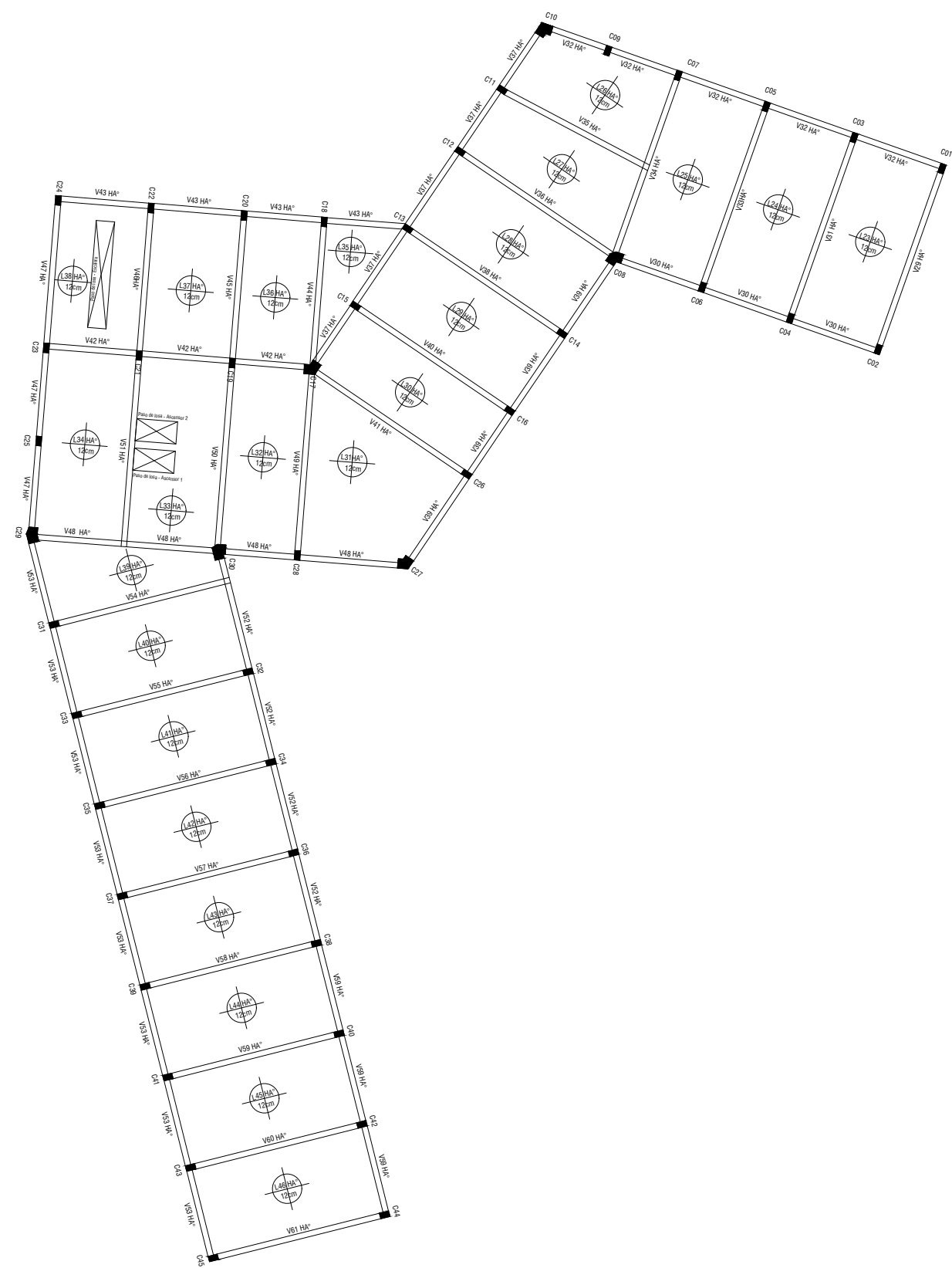
PLANTA DE ESTRUCTURA SOBRE P.A. - Esc. 1.500
