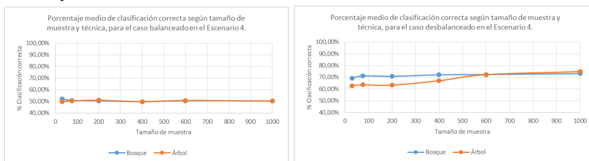
Figura 4: Porcentaje de clasificación correcta en Escenario 4 según técnica, tamaño de muestra y caso.
