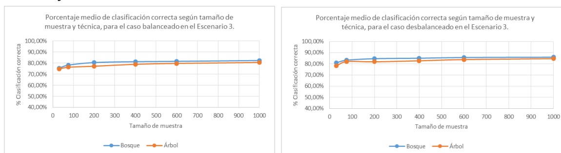
Figura 3: Porcentaje de clasificación correcta en Escenario 3 según técnica, tamaño de muestra y caso.
