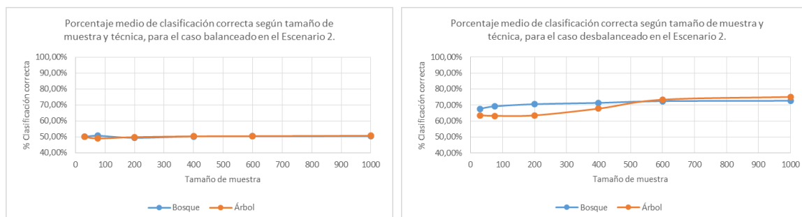
Figura 2: Porcentaje de clasificación correcta en Escenario 2 según técnica, tamaño de muestra y caso.
