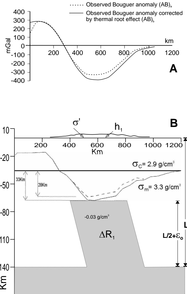
Figure 6. A: Regional observed Bouguer anomaly on 22^\circ\text{S} latitude and regional observed Bouguer anomaly corrected by the gravimetric effect due to the lithospheric thermal root; B: Crustal thicknesses corresponding to Models 1 and 2 (see Fig. 1A-B). Figura 6. A: Anomalia regional de Bouguer observada en latitud 22^\circ\text{S} y anomalia regional de Bouguer corregida por el efecto gravimetrico de la raiz térmica litosférica; B: Espesores corticales correspondientes a los Modelos 1 y 2 (véase Fig. 1A-B).
