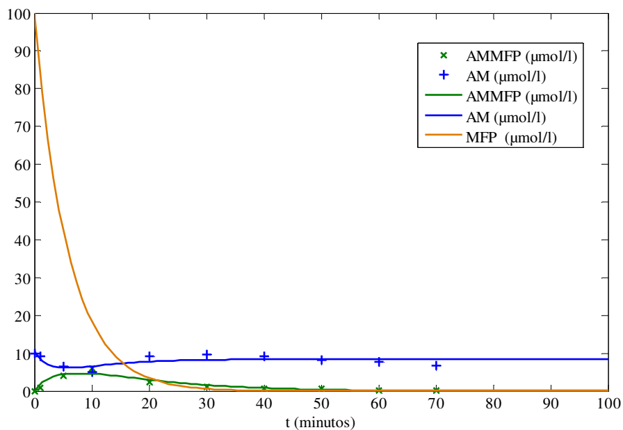
Ilustración 39: Resultados gráficos de la estimación de parámetros utilizando mediciones de AM y AMMFP. Las cruces representan los datos experimentales.
